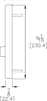
侧面图
