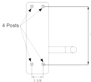
背面图
