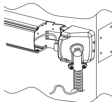
FCA/FCV 柔性导管端帽准备工作
