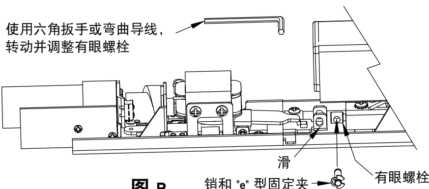
图 A 螺栓位置 (仅限边缘)
