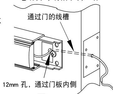
电动合叶端帽准备工作
