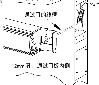
电源转换端帽准备工作
