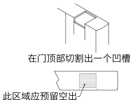
插销安装示意图
